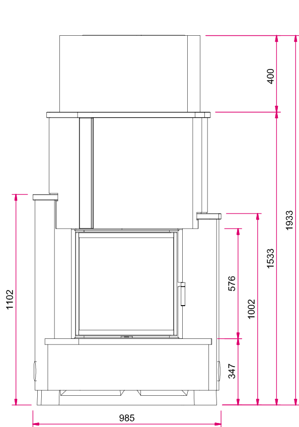
Frontansicht
