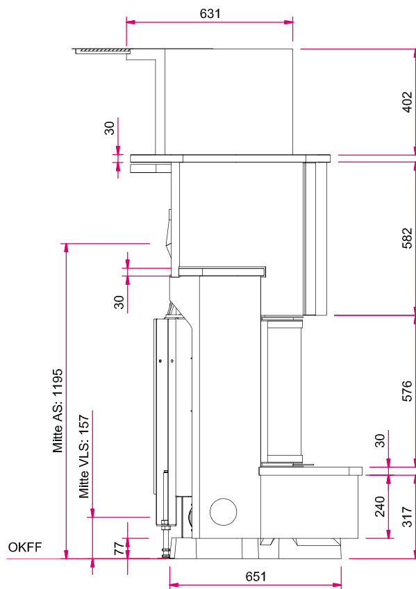
Seitenansicht
