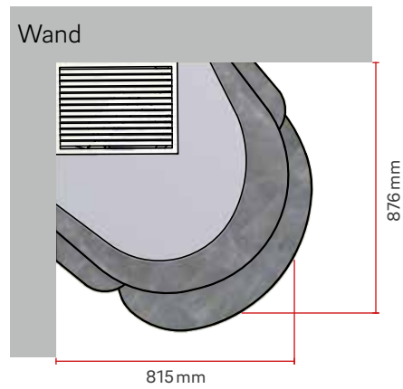
Estrichaussparung (Für die Estrichaussparung ist die beigelegte Schablone zu verwenden!)
